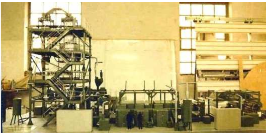
Modello di Macchina per cellophan-scala 1/10-mt.4
